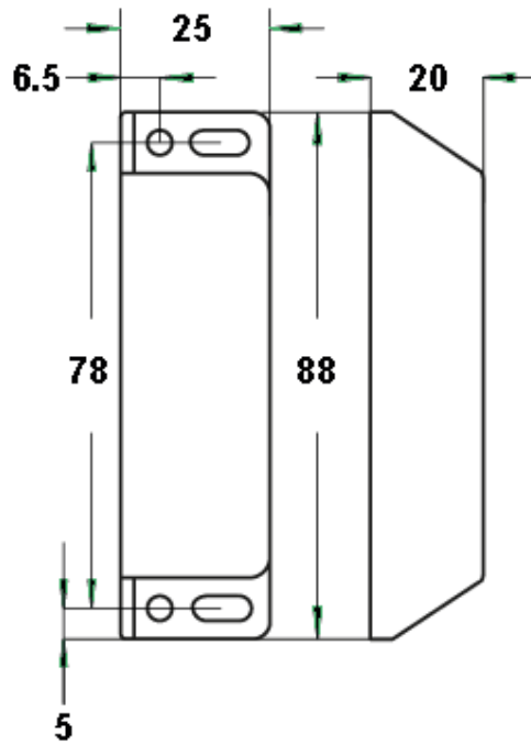
OSSG ACTUATOR
