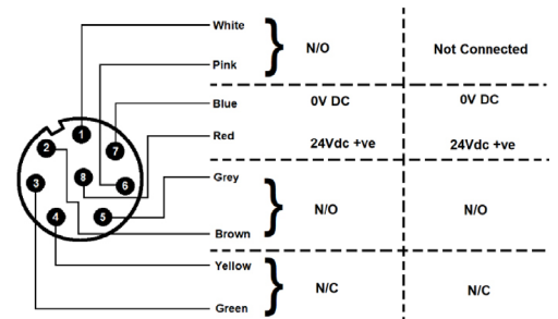
HEX21-LQD 2NO + 1NC
